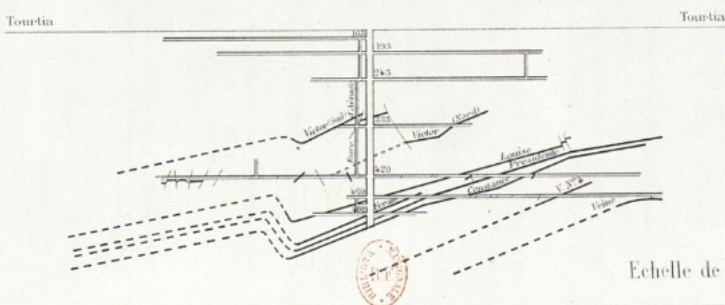
Fosse N°2. COUPE SUIVANT LA LIGNE C.D. DU PLAN.
